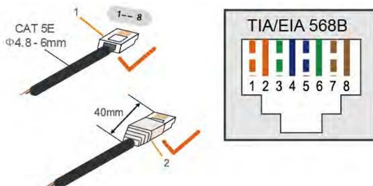
1: Fiche RJ45
