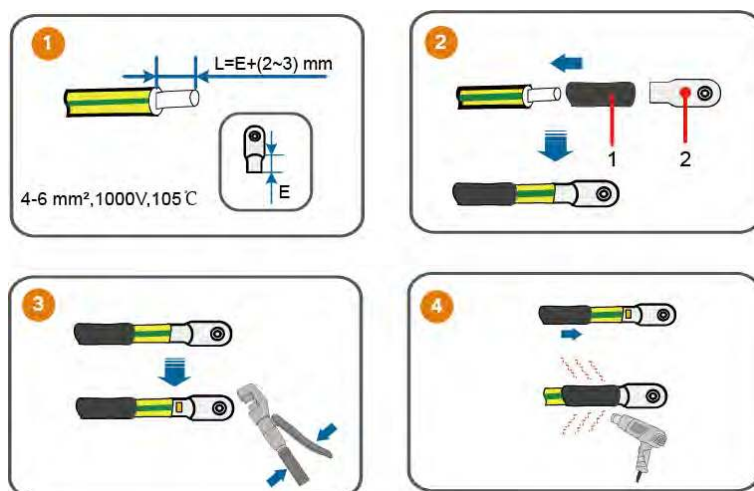
(1) Gaine thermorétractable
